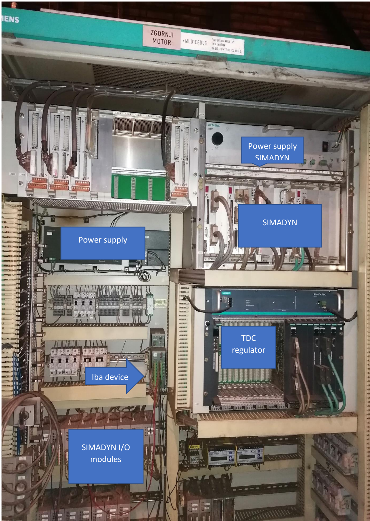
Slika 4 - Regulator for TOP motor
