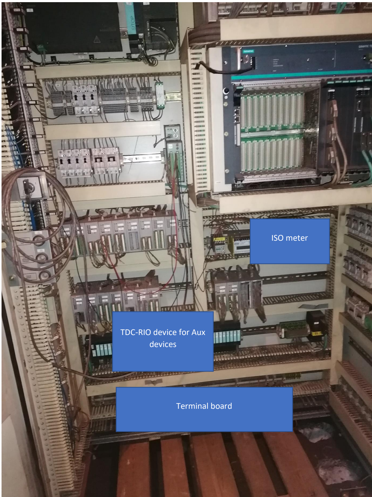
Slika 5 Regulator for TOP motor
